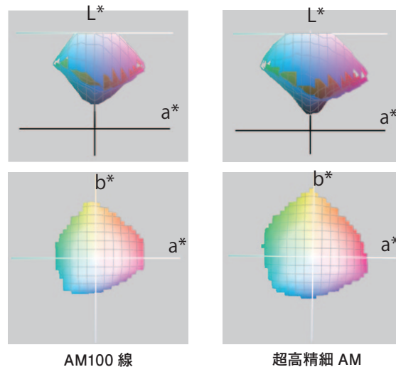
色域を示すガマツ図
